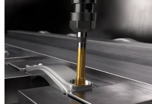
CoroTap™ 400
