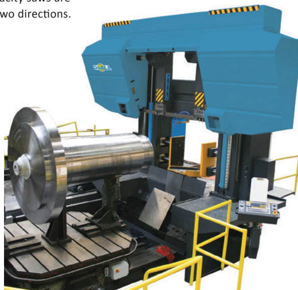
DC-1600CNC Portal
